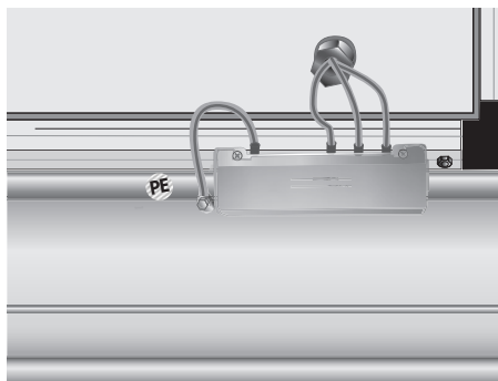
Potenzialausgleichsschiene
