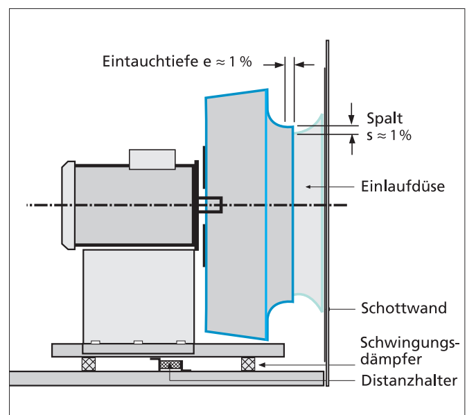
ab Ventilator-Baugröße 355
