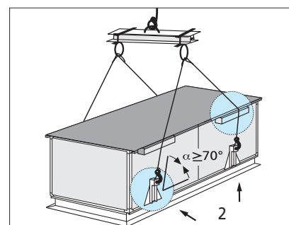
Baustellentransport mit Kran bei Gerätemodulen mit Grundrahmen
