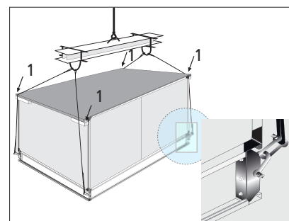
Baustellentransport mit Kran bei Gerätemodulen ohne Grundrahmen
