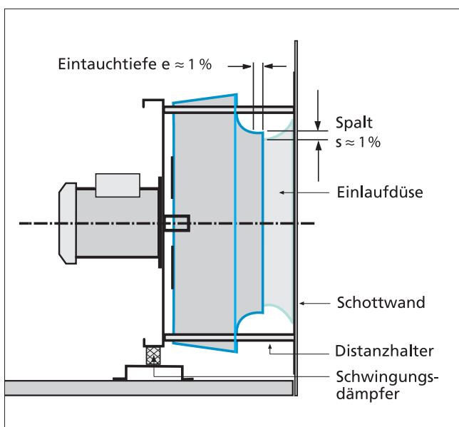
bis Ventilator-Baugröße 315
