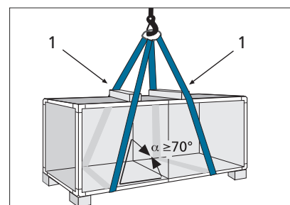
Baustellentransport mit Kran bei Gerätemodulen ohne Grundrahmen
